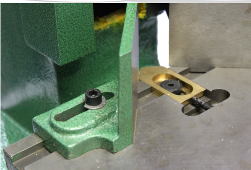
Contra fabricada en bronce, que permite exactitud
